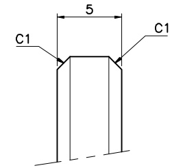
DETAIL-"A" 테두리면 면취 가공할 것
